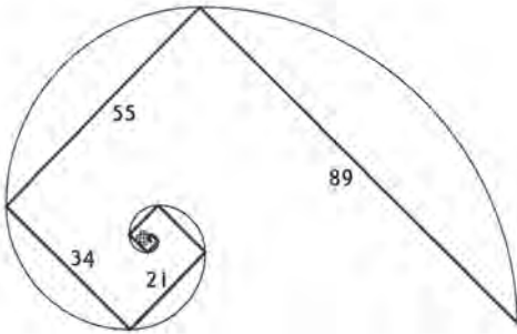
Abb. 28 Fibonacci-Spirale
